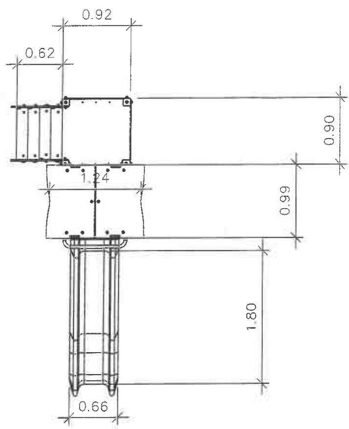
ESQUEMA TIPO
