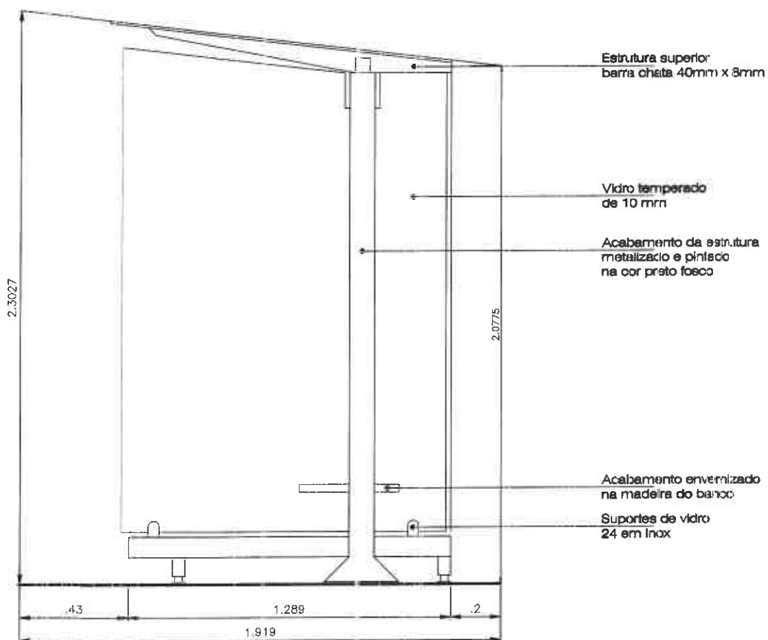
VISTA LATERAL
